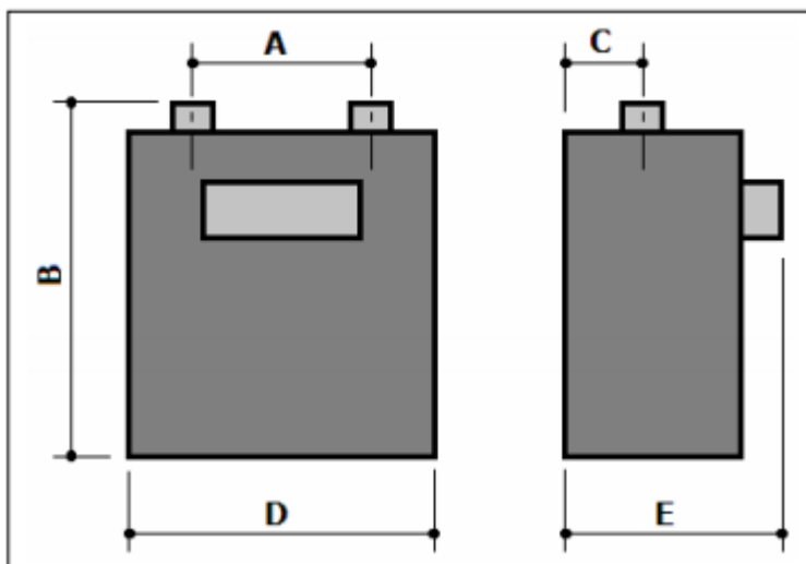
Figura 1: Dimensões do medidores
