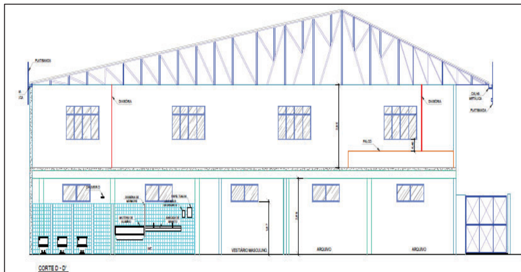
Imagem 2 - Corte lateral da planta da sede da CIGÁS
