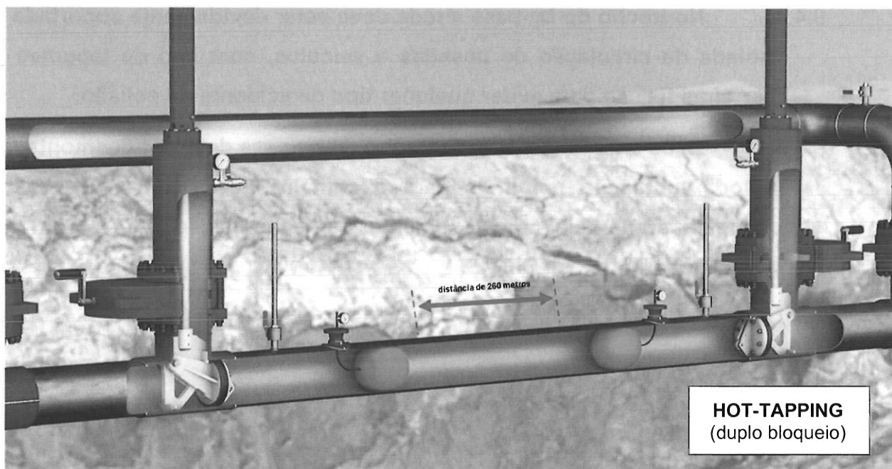
Figura 2 – Desenho esquemático do processo de hot-tapping.
