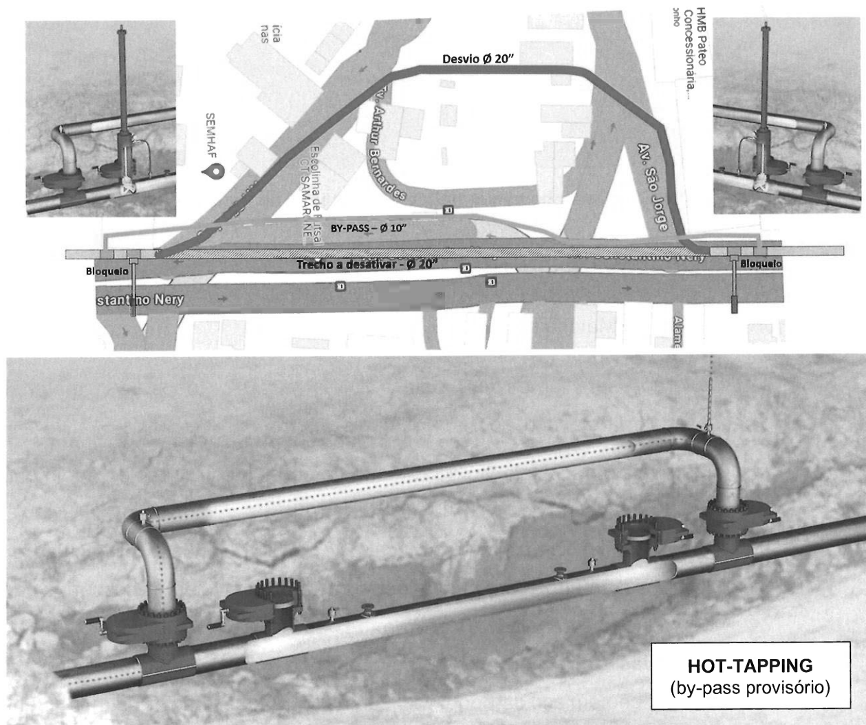
Figura 2 – Desenho esquemático do processo de hot-tapping.
